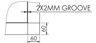
A-A SECTION
